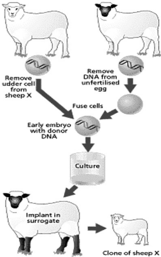
आकृती ४. क्लोनिंगने डॉली केली
