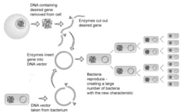
आकृती ३. वाहक विषाणू वापरून जंतूकडून प्रथिन बनवून घेणं
