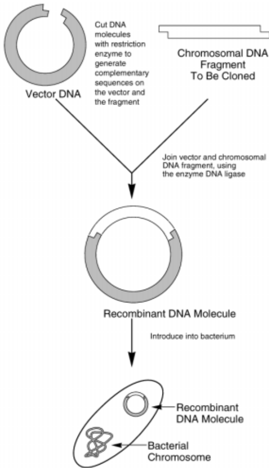
आकृती १. जनुकांची तोड-जोड
