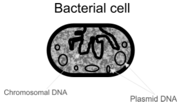
आकृती २. प्लाझ्मिड्स
